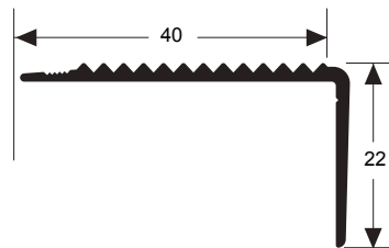
AB-129 0,252 kg/m
