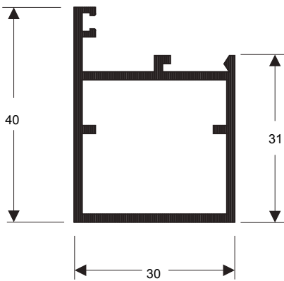
P-084 0,528 kg/m
