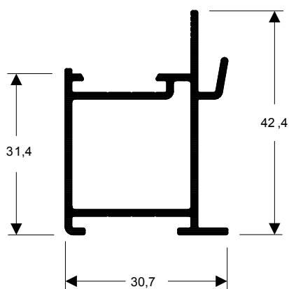
TMS-040 0,476 kg/m
