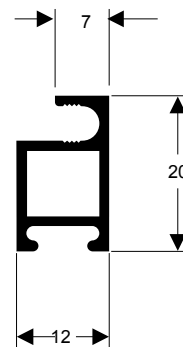
A-058 0,201 kg/m
