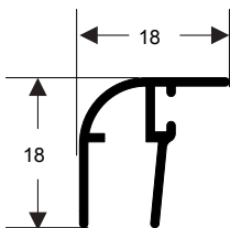
TMB-102 0,152 kg/m
