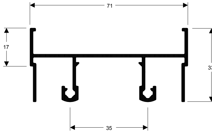
TMS-001 0,740 kg/m
