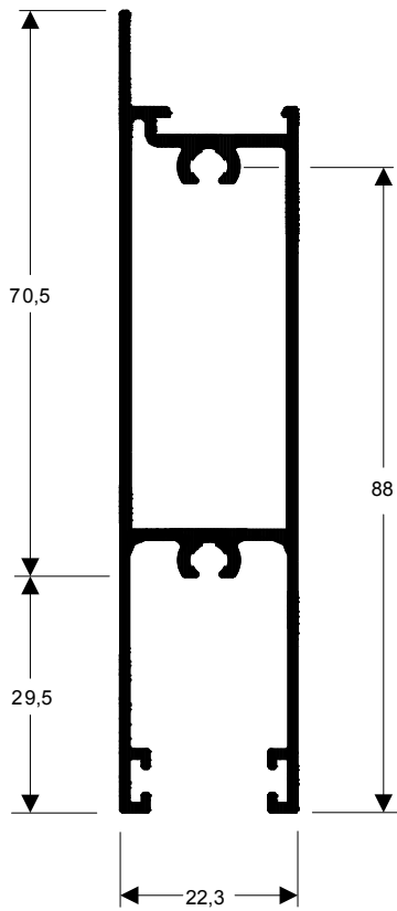
TMS-225 0,997 kg/m
