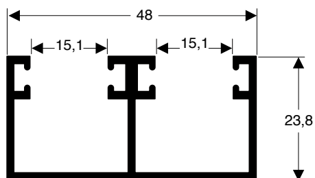
DP-011 0,547 kg/m
