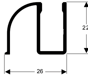
TMB-116 0,263 kg/m
