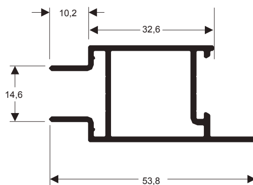
TMS-192 0,517 kg/m
