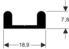
TMR-837 0,195 kg/m
