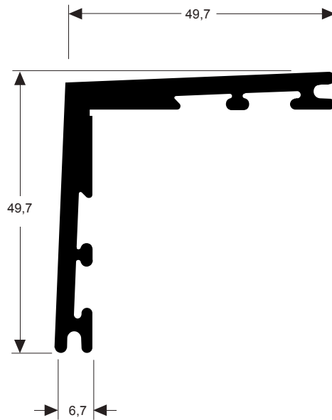
CL-006 0,997 kg/m
