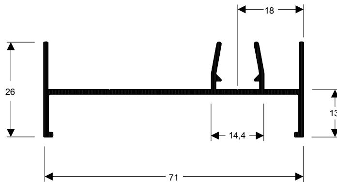
TMS-003 0,493 kg/m
