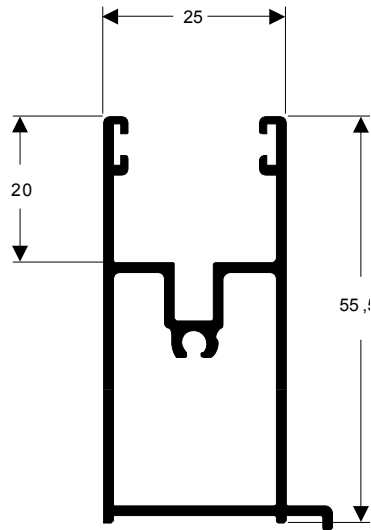
TMN-007 0,715 kg/m
