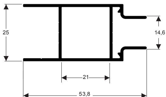
TMS-191 0,542 kg/m
