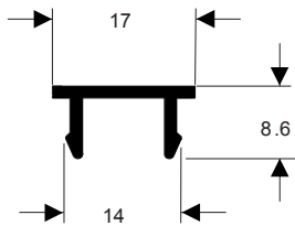
U-491 0,095 kg/m
