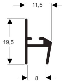
TMB-081A 0,130 kg/m
