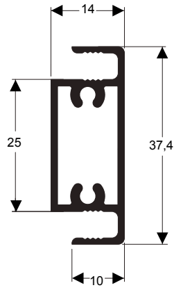
TMR-743 0,405 kg/m
