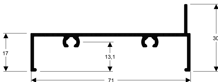
TMS-004 0,520 kg/m
