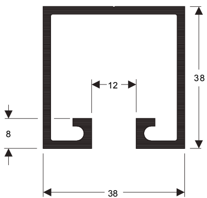
U-990 0,750 kg/m
