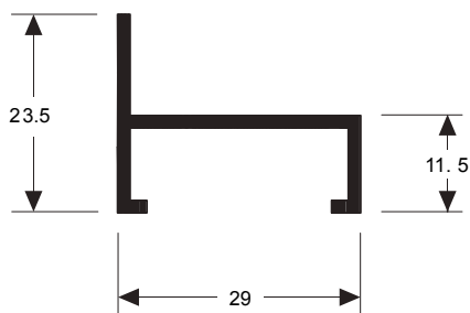
Y-120 0,222 kg/m
