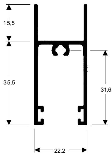
TMS-187 0,509 kg/m
