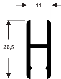
TMR-835 0,320 kg/m
