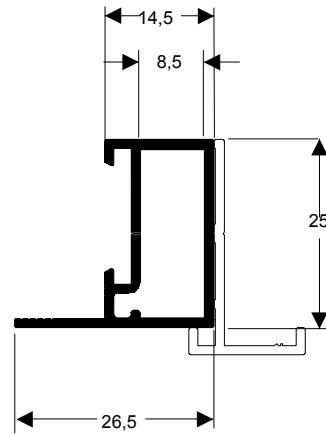
TMS-096
