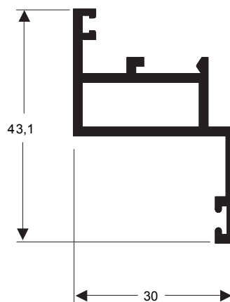
P-145 0,434 kg/m
