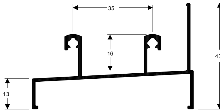
TMS-002 0,493 kg/m
