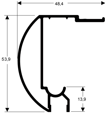
TMR-845 0,585 kg/m
