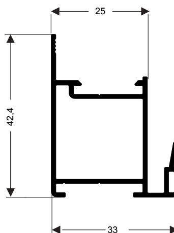
TMS-041 0,485 kg/m
