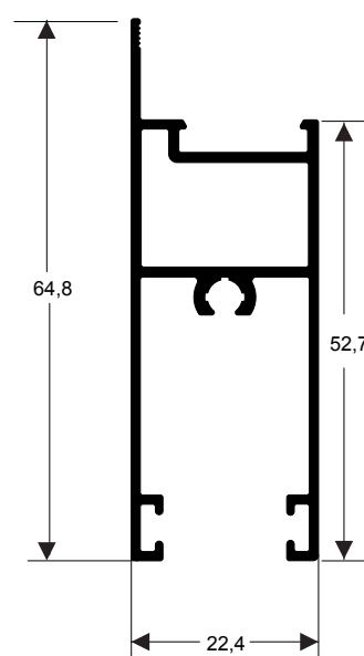
TMS-246 0,593 kg/m
