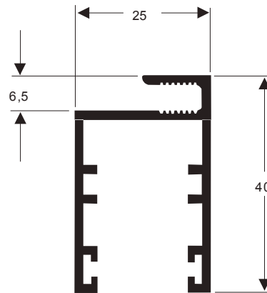
Y-312 0,512 g/m
