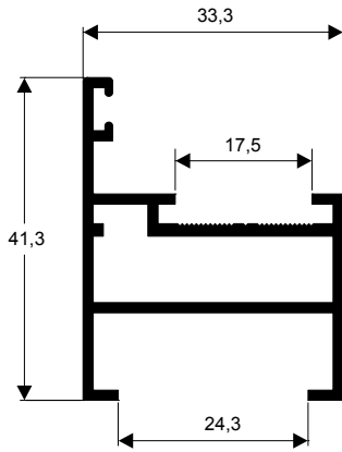
TMS-279 0,552 kg/m
