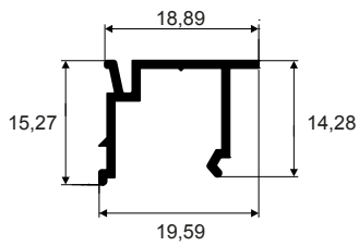
TMS-203 0,130 kg/m
