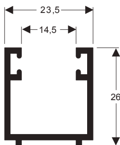
U-1108 0,358 kg/m
