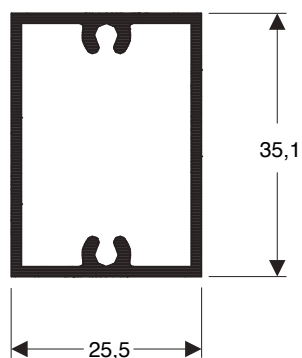
D-055 0,504 kg/m
