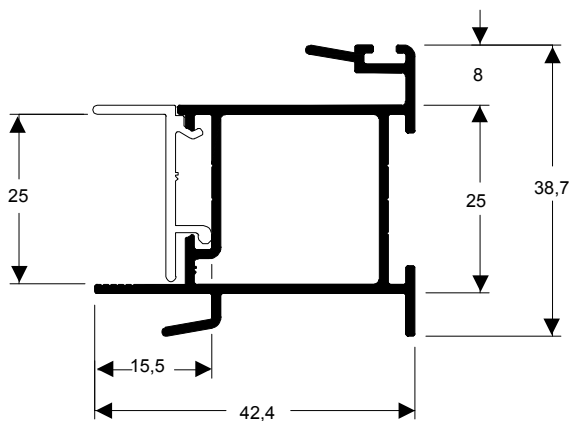
TMS-042 0,561 kg/m
