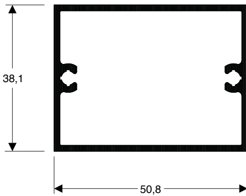
D-103 0,770 kg/m
