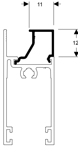
TMS-102 0,111 kg/m
