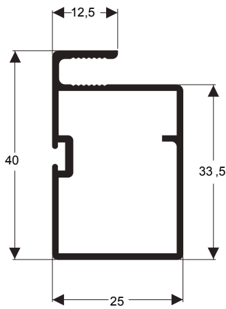
P-227 0,463 kg/m
