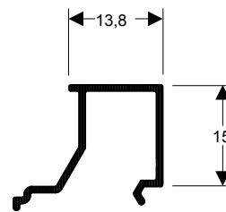
TMS-103 0,141 kg/m
