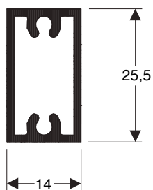
D-082 0,320 kg/m
