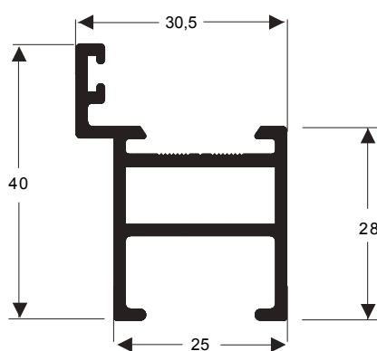
P-412 0,537 kg/m
