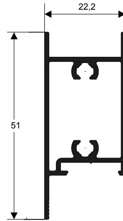
TMS-110 0,534 kg/m
