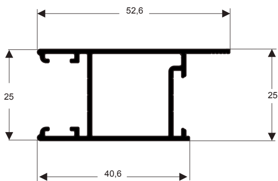
TMS-039 0,488 kg/m
