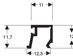
U-522 0,092 kg/m
