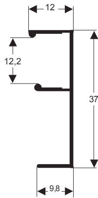
MP-347 0,184 kg/m
