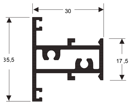
P-075 0,550 kg/m
