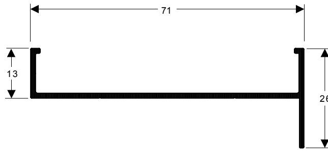
TMS-007 0,386 kg/m
