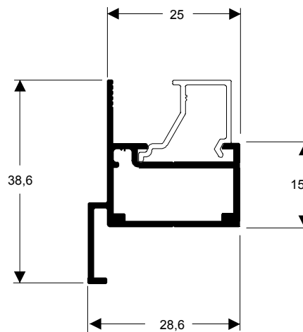
TMS-097
