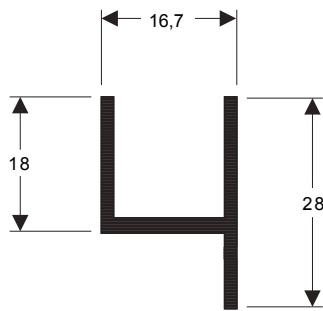
Y-107 0,184 kg/m
