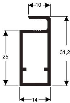
TMR-742 0,315 kg/m
