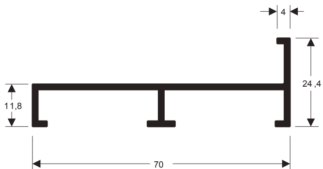
E-277 0,447 kg/m
