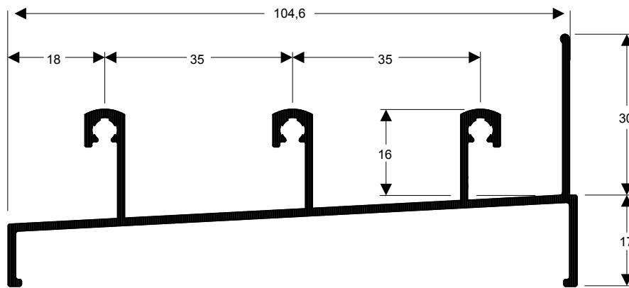
TMS-011 0,940 kg/m
