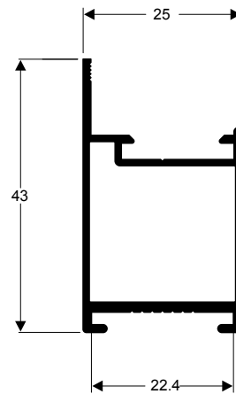
TMS-120 0,466 kg/m
