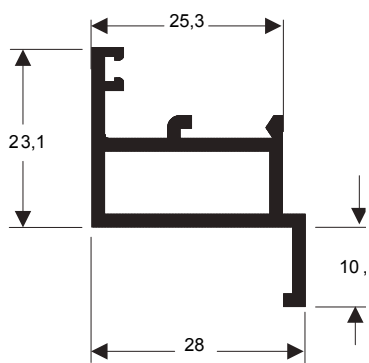
P-166 0,376 kg/m
