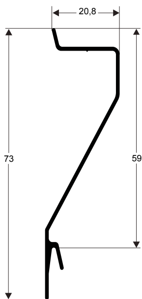
Z-203P 0,322 kg/m
