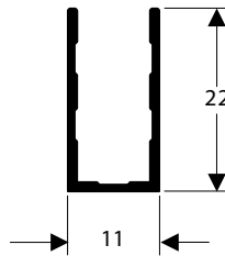
DP-001 0,141 kg/m
