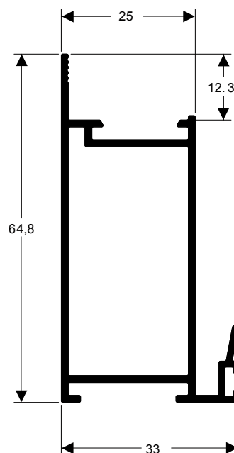
TMS-242 0,710 kg/m
