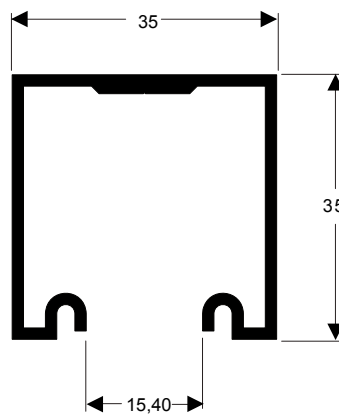
U-1098 0,569 kg/m
