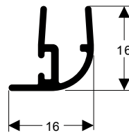
TMR-793 0,141 kg/m
