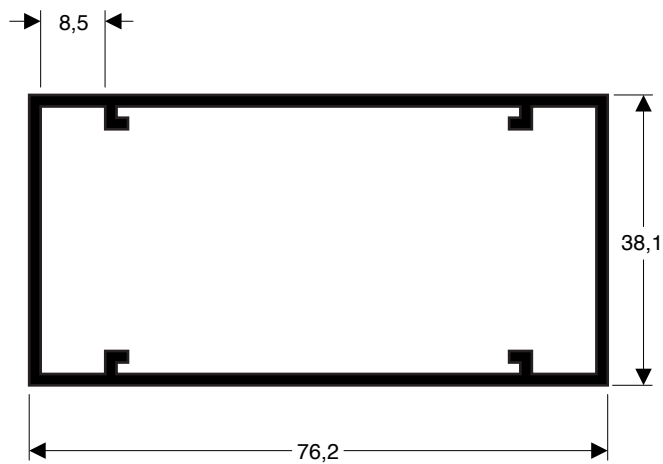
D-069 0,900 kg/m
