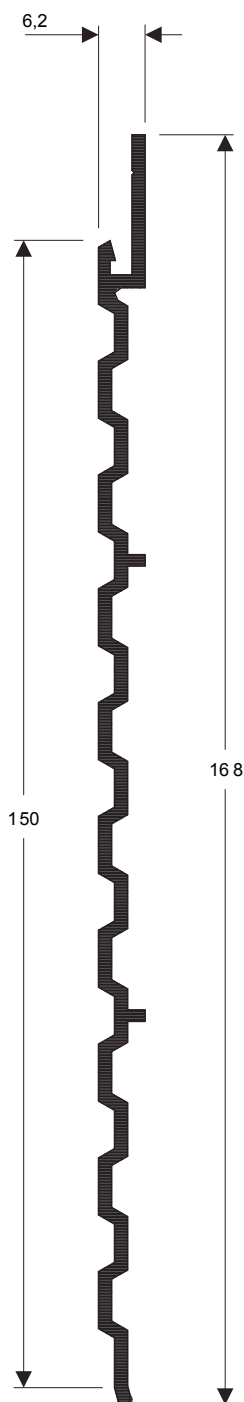
Y-355 0,688 kg/m
