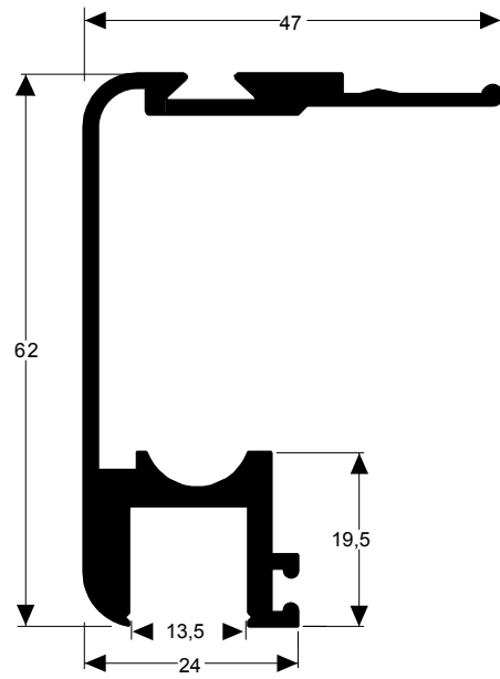
L-713A 0,957 kg/m
