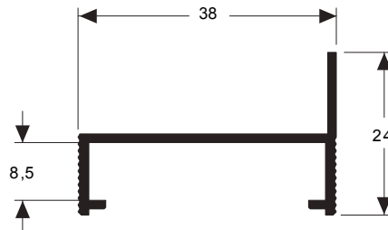
CM-060 0,241 kg/m
