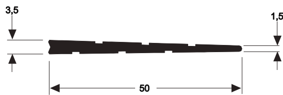
CL-011 0,317 kg/m
