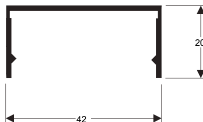
U-621 0,265 kg/m
