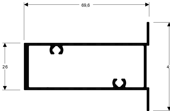
TMS-009 0,893 kg/m
