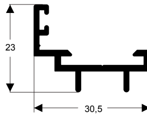
L-715 0,279 kg/m
