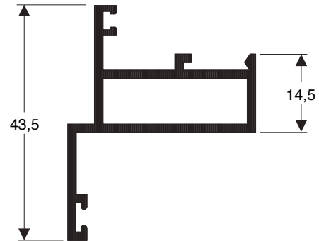
P-120 0,531 kg/m
