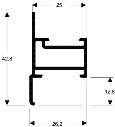
TMS-081
