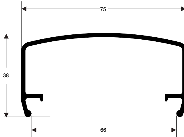
39-081 0,772 kg/m
