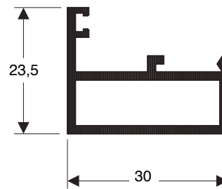
P-064 0,383 kg/m
