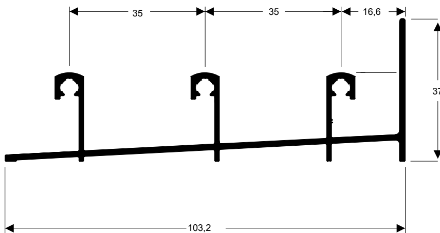
TMS-230 0,940 kg/m
