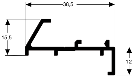
Z-063 0,308 kg/m
