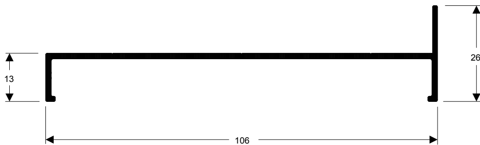
TMS-012 0,542 kg/m
