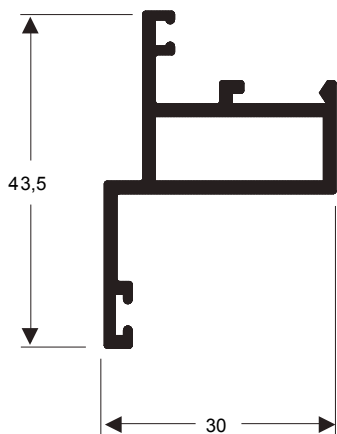
P-146 0,401 kg/m
