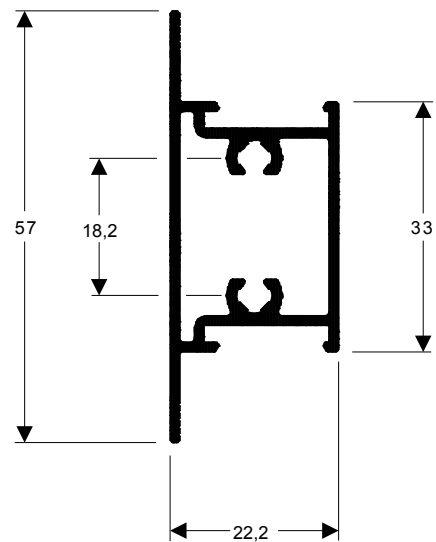
TMS-227 0,556 kg/m
