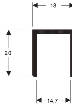
U-398 0,249 kg/m
