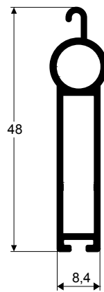
TMN-055 0,380 kg/m
