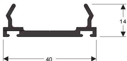
U-615 0,368 kg/m
