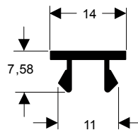
TMR-716 0,084 kg/m
