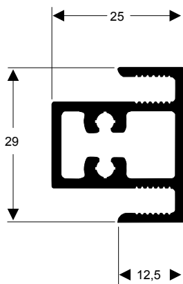
P-256 0,520 kg/m
