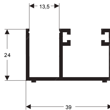
E-306 0,428 kg/m
