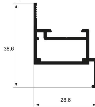
TMS-098
