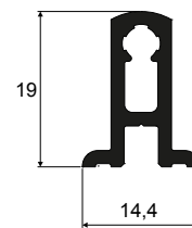
TMS-017 0,233 kg/m
