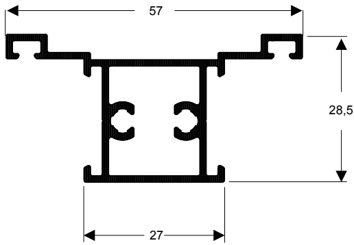
TMS-086
