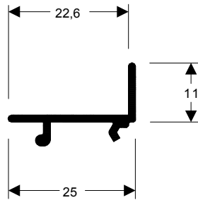
TMS-108 0,142 kg/m
