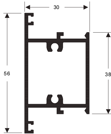
P-078 0,683 kg/m
