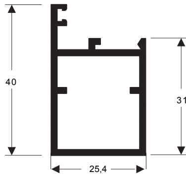
P-140 0,436 kg/m
