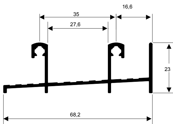
TMS-260 0,609 kg/m
