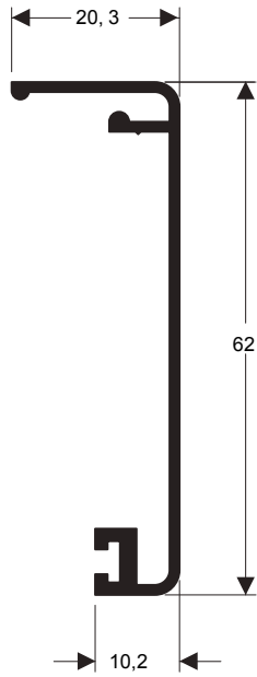
E-512A 0,380 kg/m
