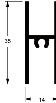
I-083 0,339 kg/m
