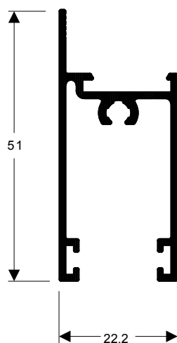
TMS-053 0,471 kg/m
