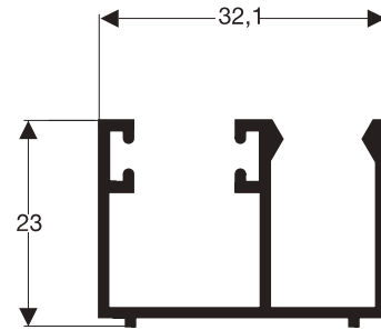
TMR-714 0,328 kg/m
