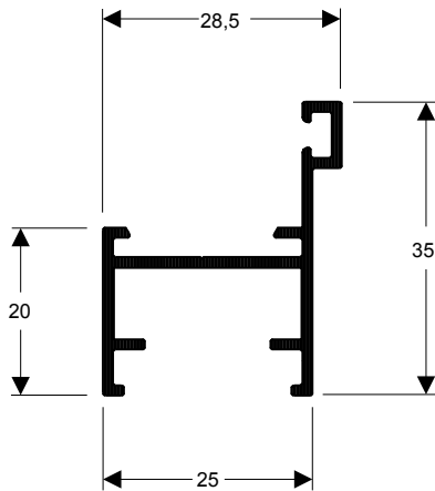
TMS-079
