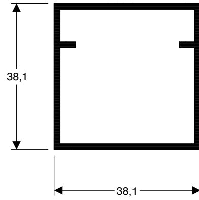
D-102 0,547 kg/m
