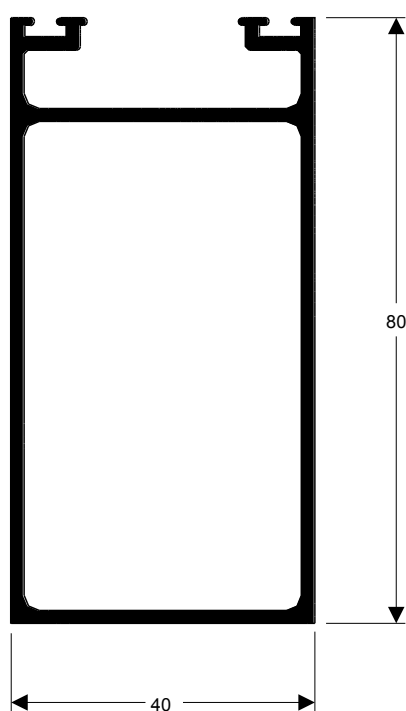
A-072 1,203 kg/m
