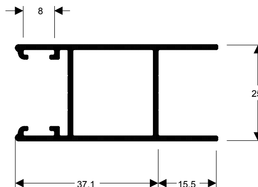
TMS-068 0,495 kg/m
