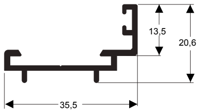
L-519 0,274 kg/m
