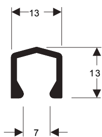
U-681 0,117 kg/m
