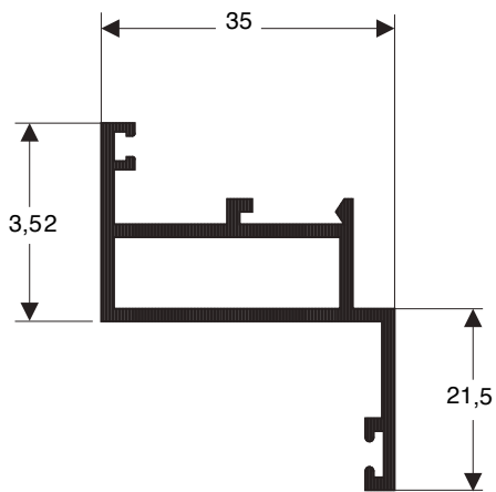
P-121 0,504 kg/m
