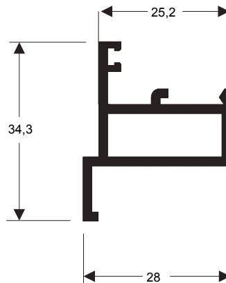
P-167 0,377 kg/m
