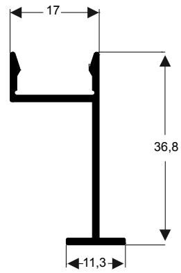
TMR-1447 0,252 kg/m
