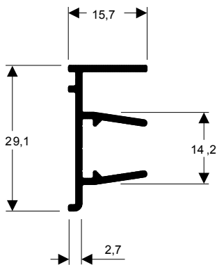
TMS-008 0,247 kg/m
