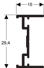
I-105 0,230 kg/m
