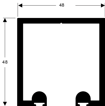
TMR-1035 1,436 kg/m
