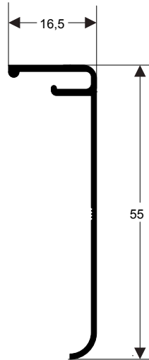
TMB-115 0,233 kg/m
