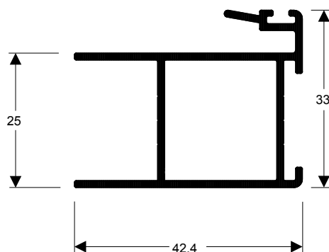
TMS-070 0,517 kg/m
