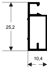
TMR-1190 0,190 kg/m
