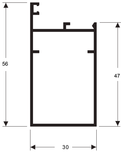
P-068 0,555 kg/m
