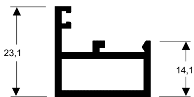
P-147 0,325 kg/m
