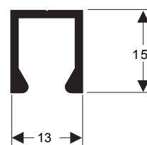
U-425 0,154 kg/m
