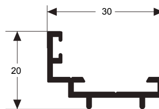
L-592 0,282 kg/m
