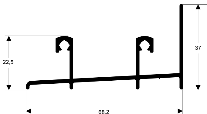
TMS-228 0,669 kg/m
