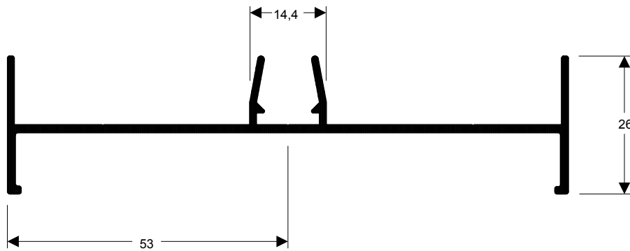
TMS-014 0,647 kg/m
