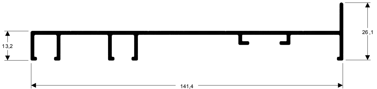
TMS-123 0,970 kg/m
