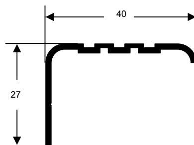
ME-013 0,266 kg/m
