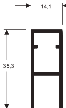
A-022 0,317 kg/m
