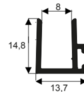
TMR-790 0,157 kg/m
