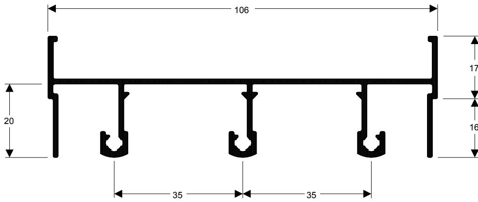
TMS-010 0,989 kg/m
