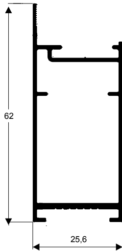
TMS-111 0,615 kg/m
