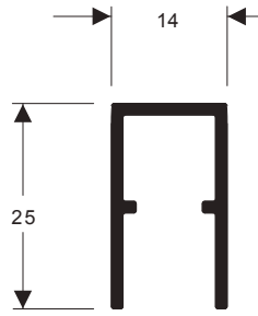
U-396 0,239 kg/m
