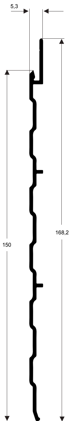
Y-429 0,632 kg/m
