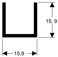
U-509 0,192 kg/m
