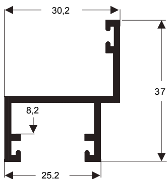
Y-126 0,347 kg/m
