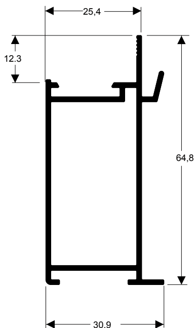
TMS-243 0,710 kg/m
