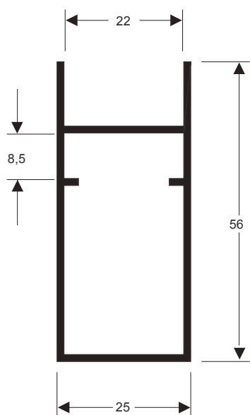
A-194 0,572 kg/m
