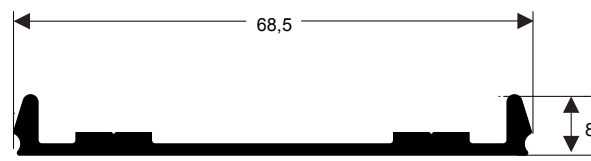
U-1092 0,442 kg/m
