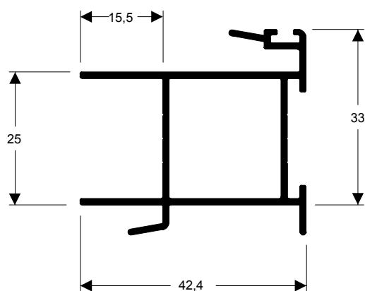
TMS-069 0,577 kg/m
