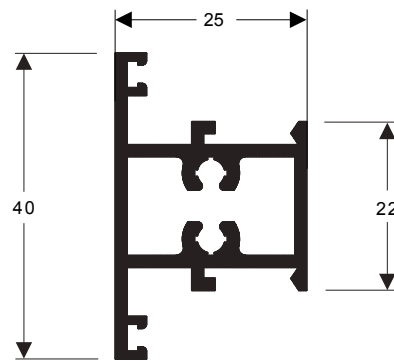
P-153 0,532 kg/m
