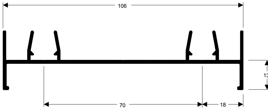
TMS-013 0,742 kg/m
