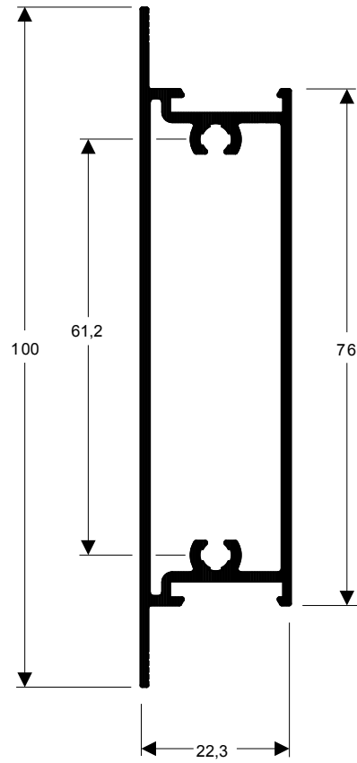
TMS-050 0,930 kg/m
