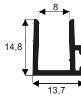
TMR-790 0,157 kg/m
